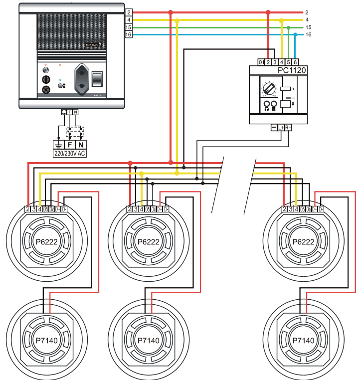
Esquema 2. 1 canal estéreo Habitación con mas de 2 plafoneras
