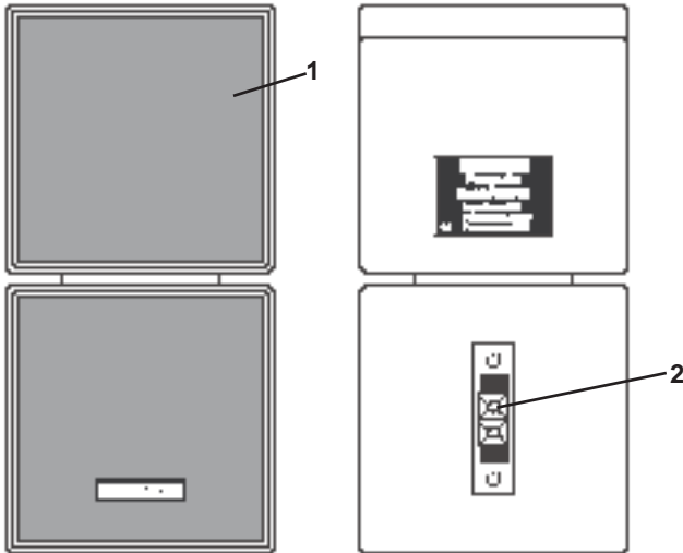
1.-Altavoz 2 1/2" ORIENTABLE 2.- Bornes de conexión
